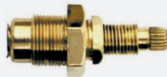
COD: 2055 - Cabezal Ph Vástago 1137 Ø 20,6 - 19 H x pulg.
